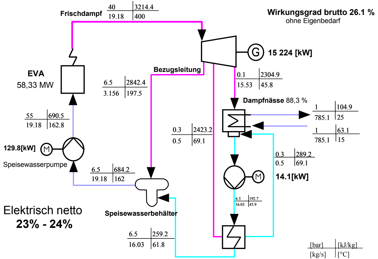
Bild 15: KPRO Schaltung Standardanlage
