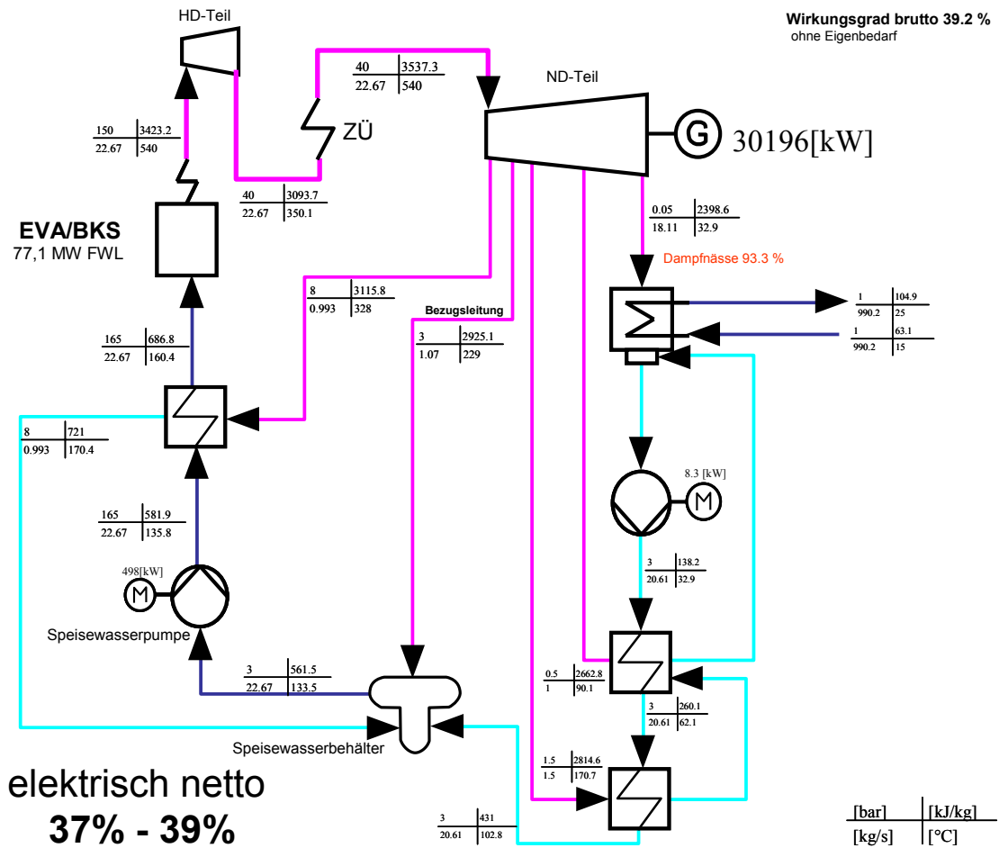
Bild 16: KPRO Schaltung BiFuelCycle-Anlage
